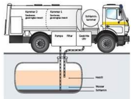
Arbeitsprinzip Tankreinigung
